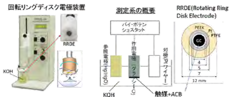
図3: 電気化学測定系の模式図
