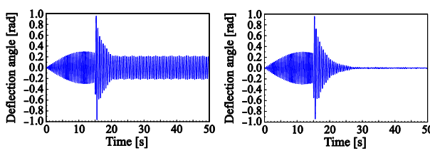
(a) 動的量子化器なし (b) 動的量子化器あり (a) : A/D 10 bit ・ D/A 6 bit ・ 動的量子化器なし (b) : A/D 6 bit ・ D/A 6 bit ・ 動的量子化器あり
