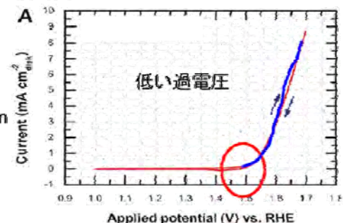
図5: 正極に触媒を添加した際の電流密度
