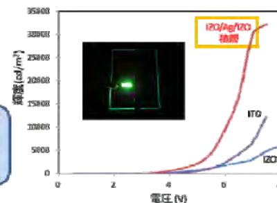
有機EL素子の発光特性
