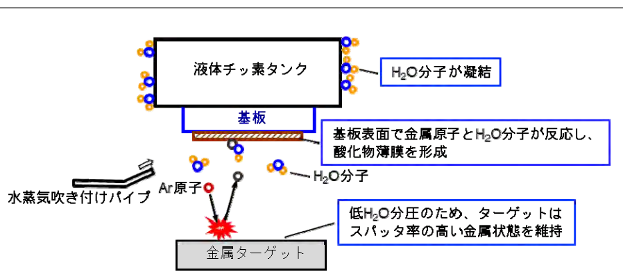
水蒸気を反応ガスに用いた高速スパッタ成膜技術の原理
