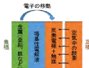
図1: 金属空気電池の概要
