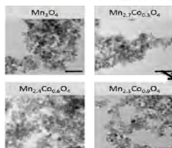
図4: 二元機能触媒(ナノ粒子)の例
