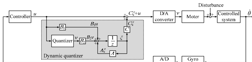
図2 動的量子化器を適用した制御系
