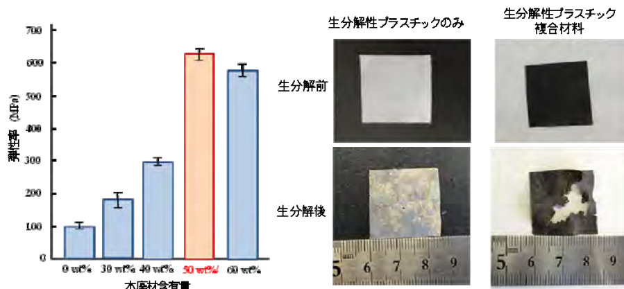
図1 木廃材含有量と弾性率の関係 図2 土中での生分解(140日)前後の写真
