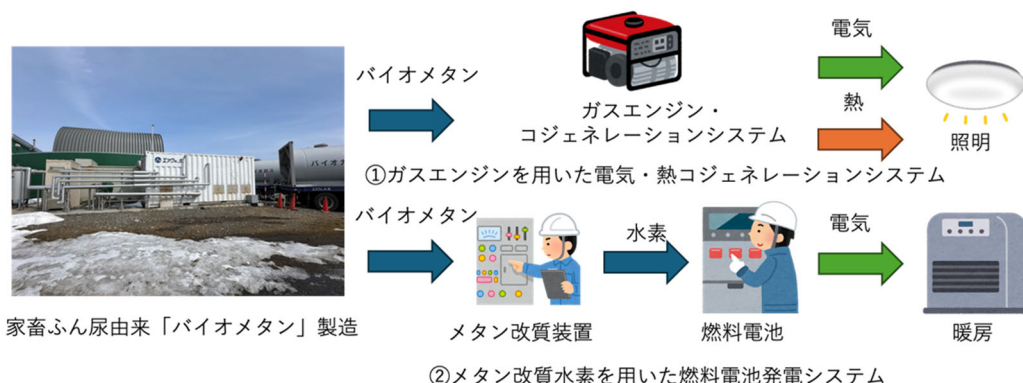
図1 バイオメタンエネルギーシステム
